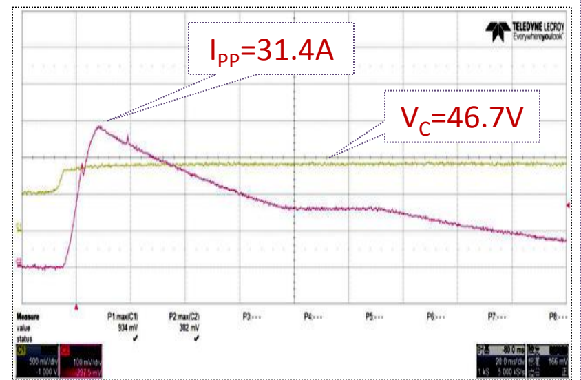
ISO16750-2 5a Test R_i=8\Omega
