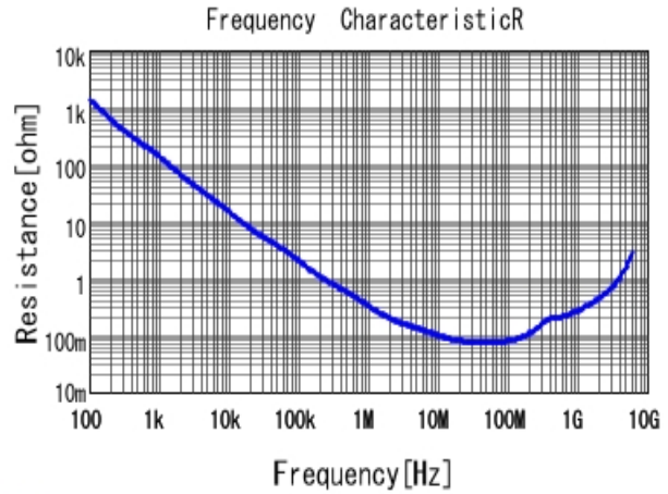
■ GRM155B31H682KA88 R DCOV, 20degC
