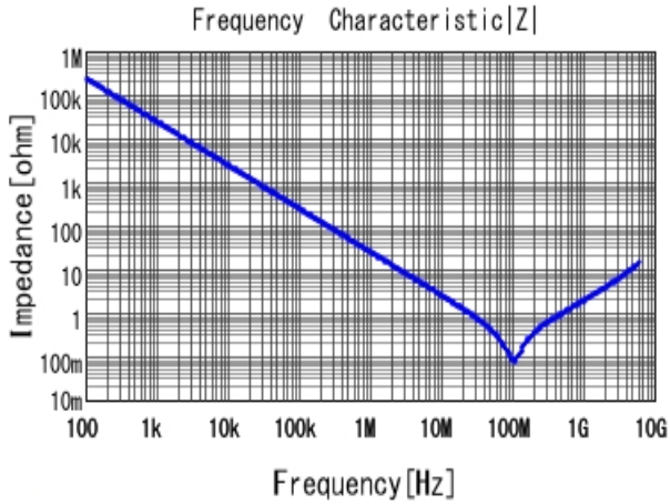
■ GRM155B31H682KA88 |Z| DCOV, 20degC
