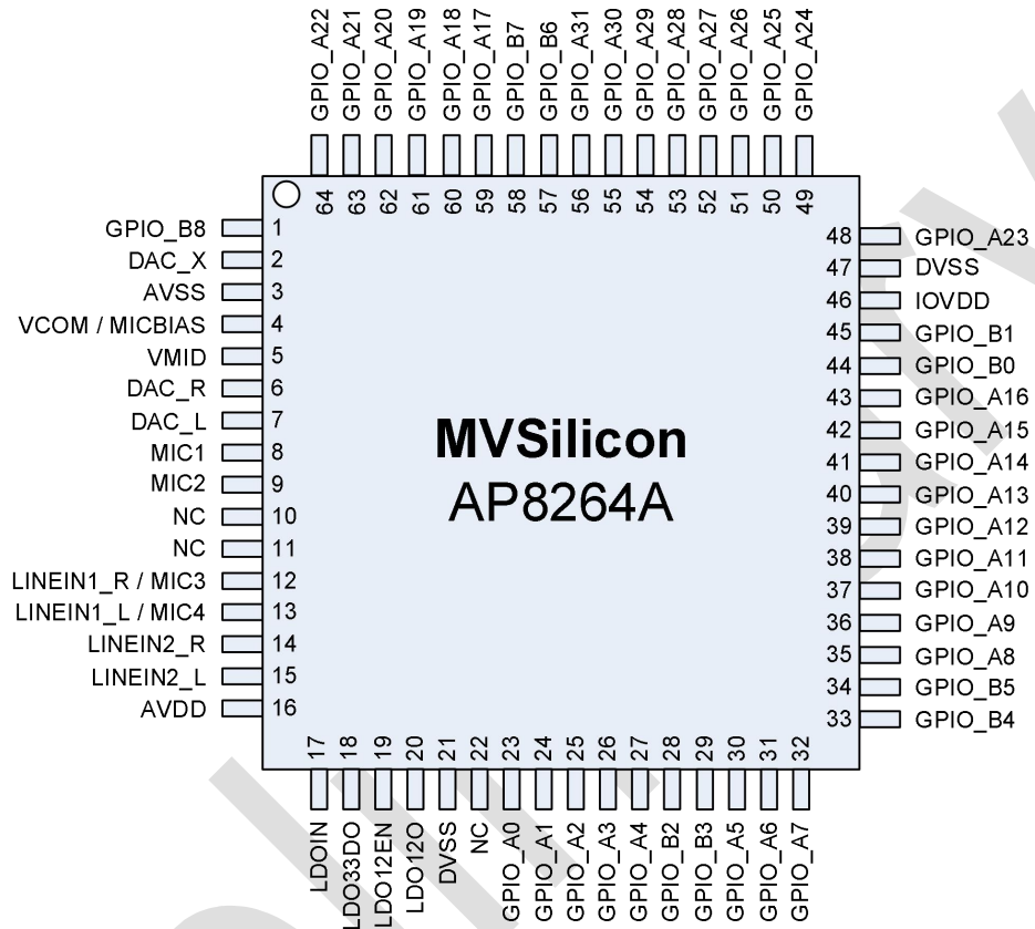
图 2. 芯片引脚定义
