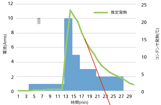
過渡電流条件/コンデンサ発熱推移
