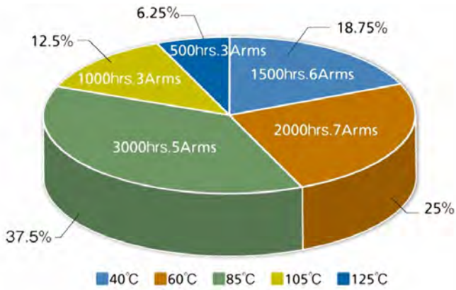
時間/周囲温度/電流 Time/Ambient Temperature/Current
